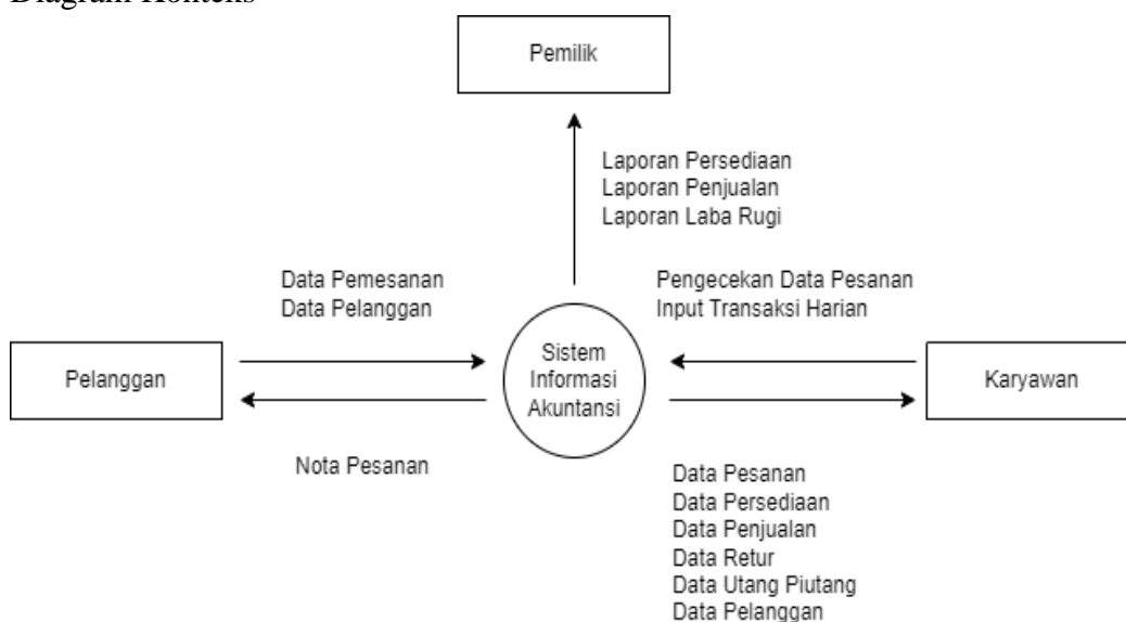
Gambar 1 Diagram Konteks
